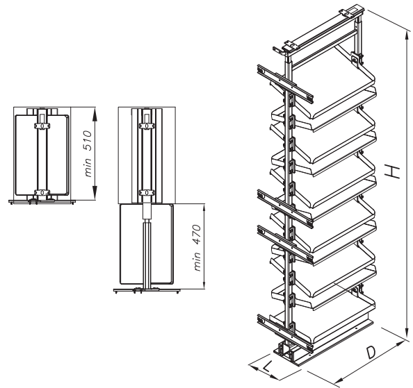
1710-1910 mm 11-półkowy / 11-shelves 1910-2110 mm 13-półkowy / 13-shelves Układ naprzemienny lub jednostronny P lub L / Alternating or single-side arrangement R or L
